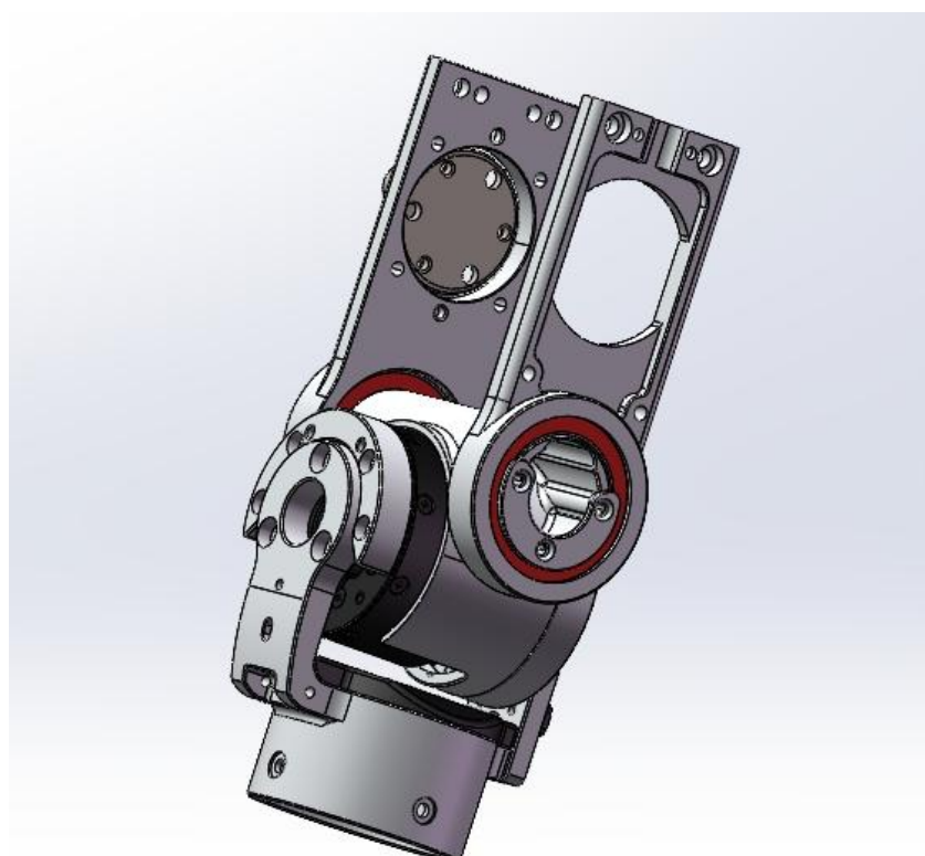
图 3 夹爪版手臂部分机械结构示意图
