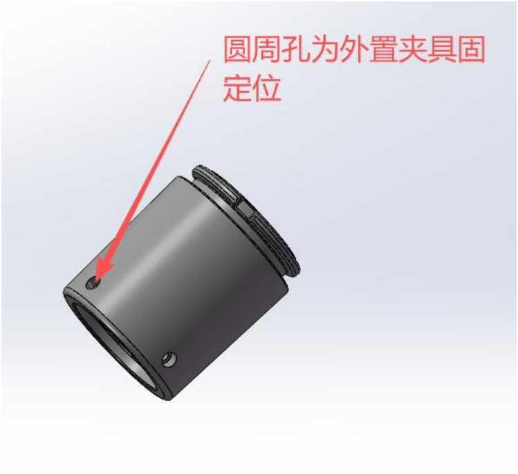
图 1 灵巧手/夹爪末端机械安装接口工程图
